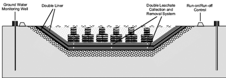
شکل شماره ۱- مقطع یک لندفیل
